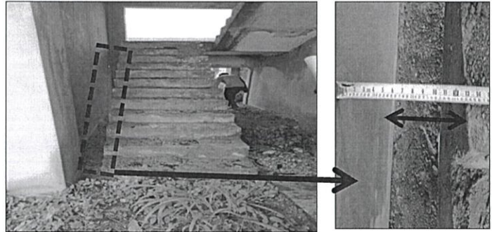
Blok Asrama Lelaki dan Perempuan - Terdapat Jurang (Gap) di Antara Tangga dan Dinding Bata Pada Semua Struktur Tangga (01.08.2018) (Sumber: Jabatan Audit Negara)
