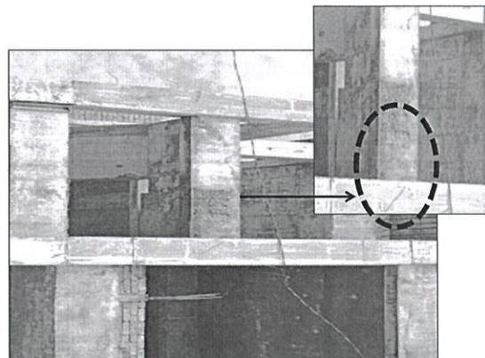
Blok Asrama Lelaki, Blok B (Akademik 1) - Terdapat Honeycomb Pada Tiang dan Rasuk (01.08.2018) (Sumber: Jabatan Audit Negara)
